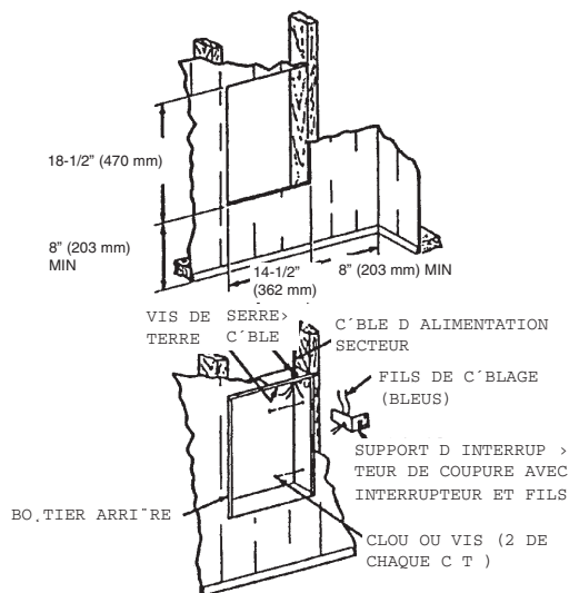
Fig. 2: Positionnement du boîtier arrière dans une construction existante
