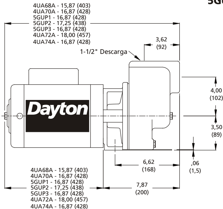
Dibujo 2 - Dimensiones (mm) pulgadas
