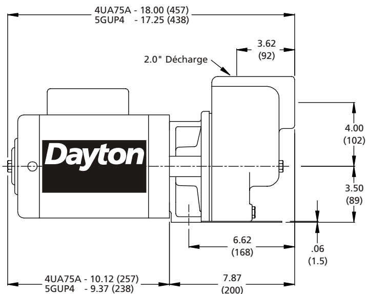
Schéma 2 - Dimensions (mm)
