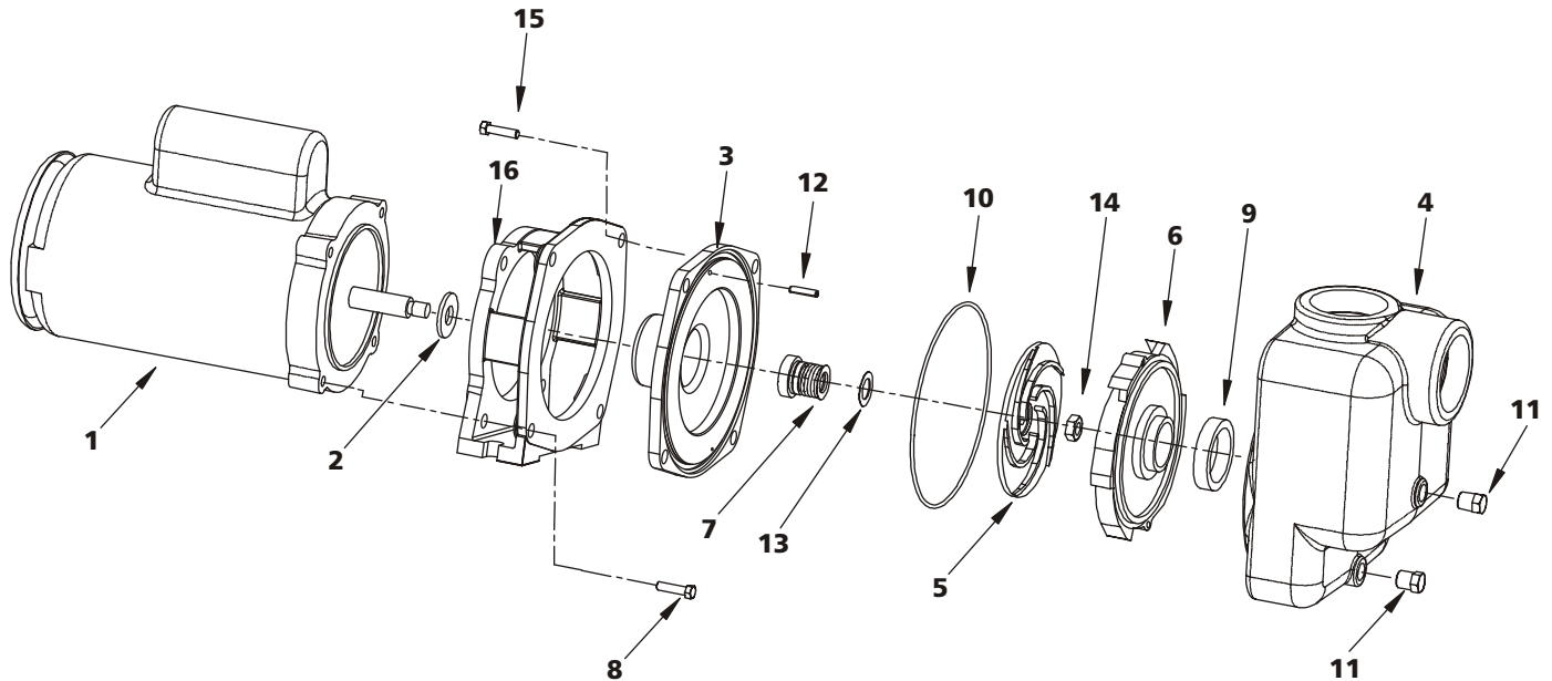
Dibujo 7 – Ilustración de piezas de reparación
