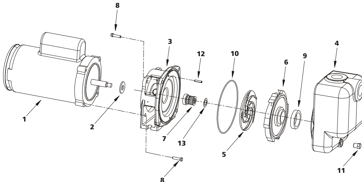
Dibujo 7 – Ilustración de piezas de reparación
