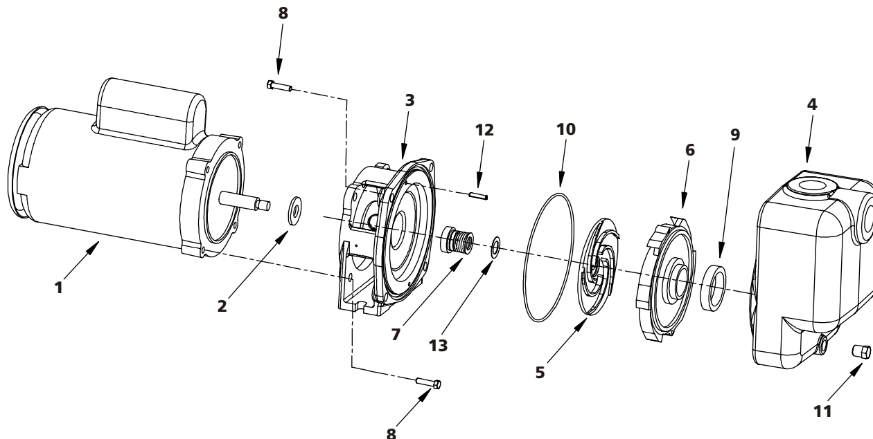
Le schéma 7 - Illustration de pièces de réparation
