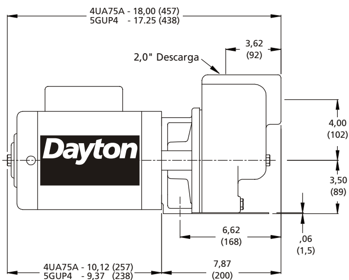
Dibujo 2 - Dimensiones (mm) pulgadas
