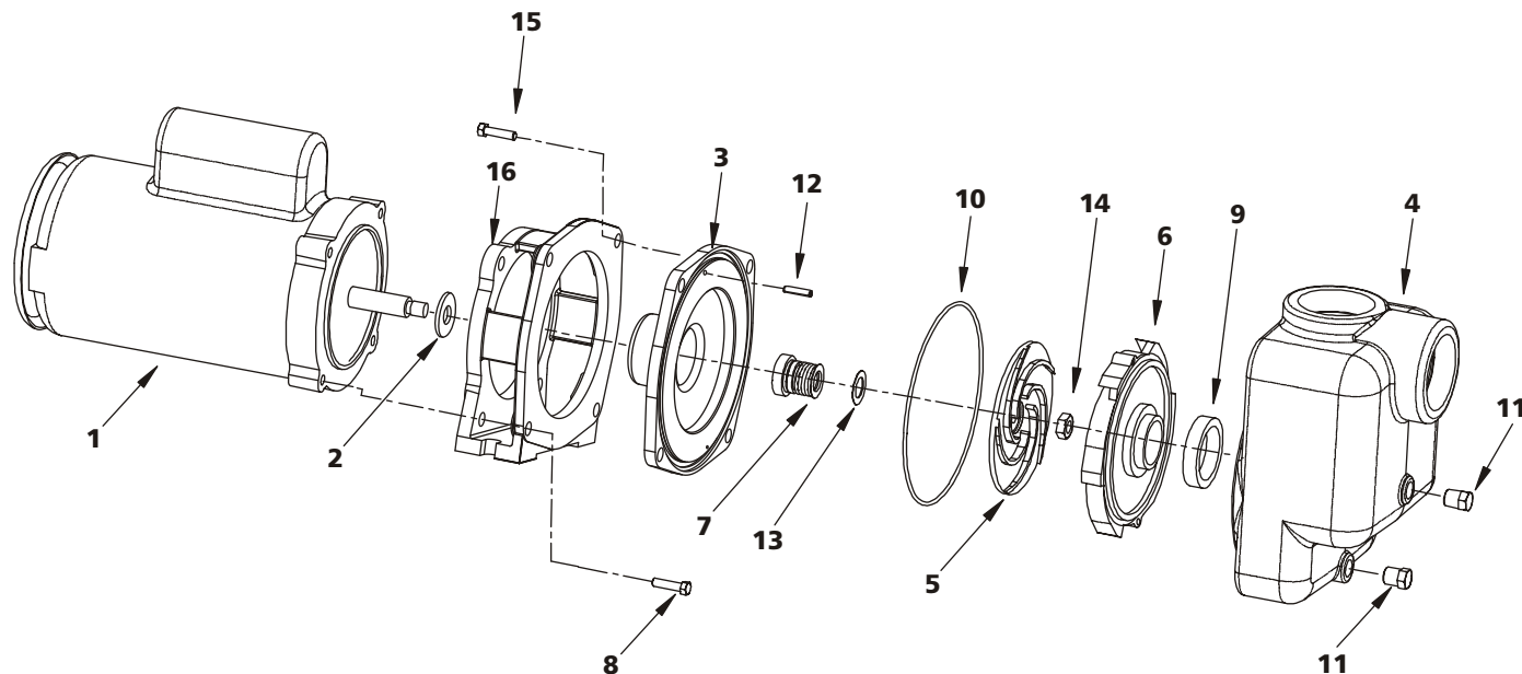
Dibujo 7 – Ilustración de piezas de reparación
