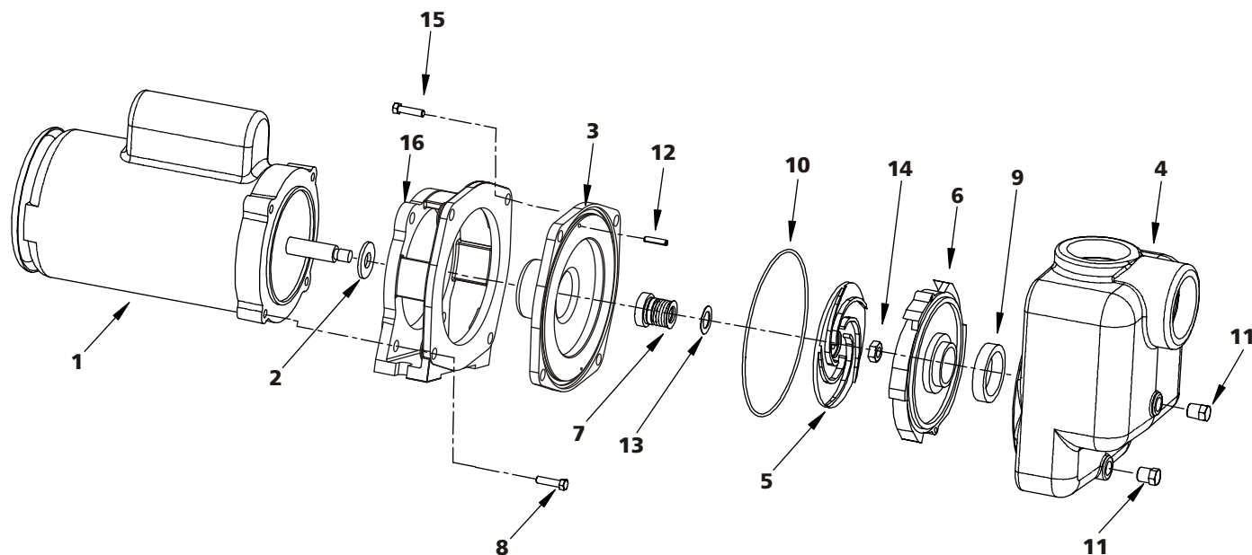
Le schéma 7 - Illustration de pièces de réparation
