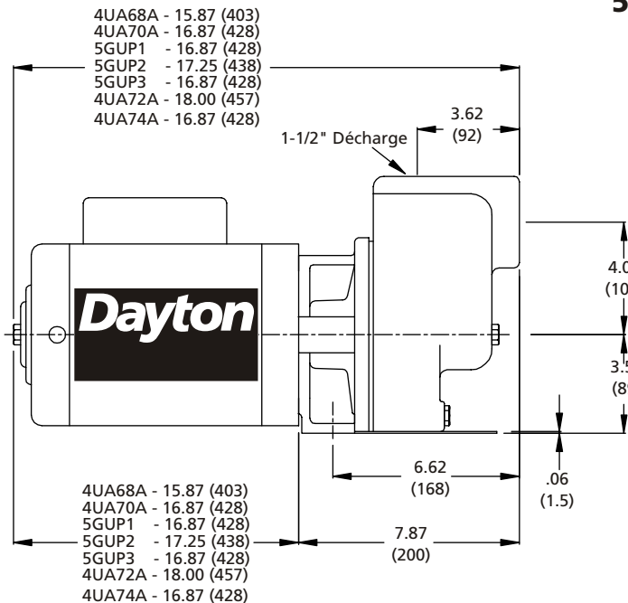
Schéma 2 - Dimensions (mm)
