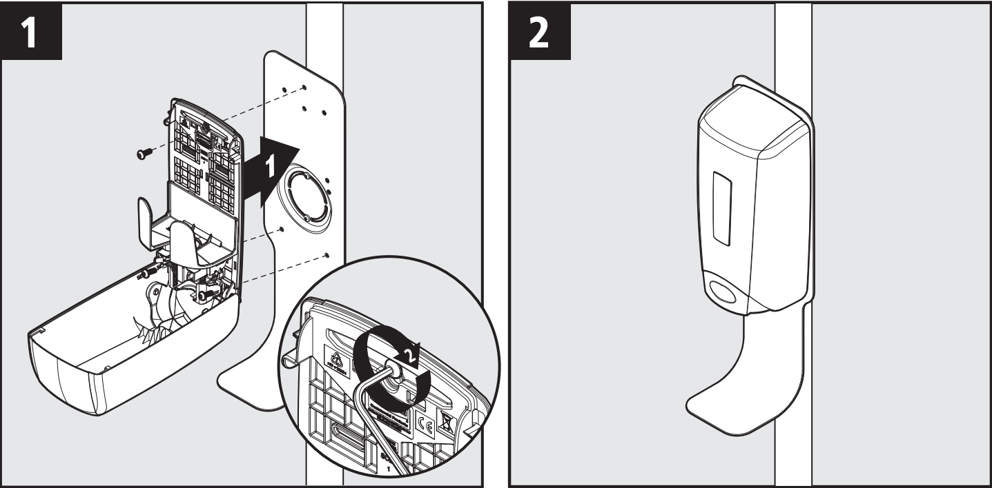
Flex™ Dispenser Installation / Instalación del dispensador Flex™ / Installation du distributeur Flex™
