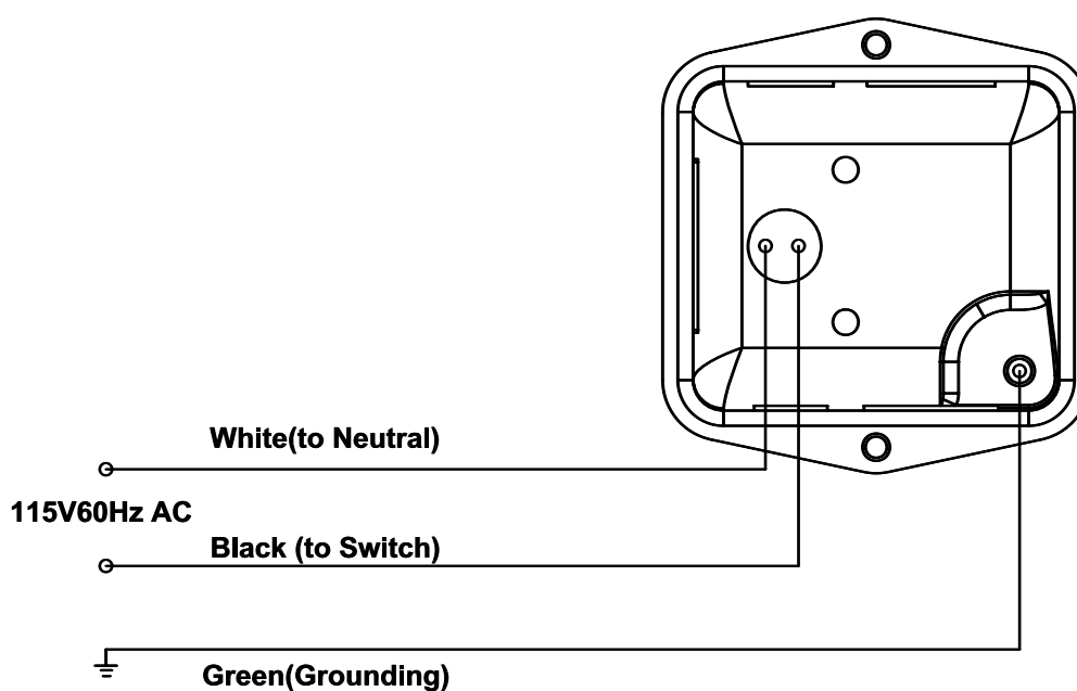
Figura 2 - Diagrama de cableado. 115 volts conexión.
